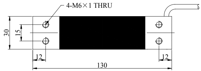
俯视图 (Top View)
