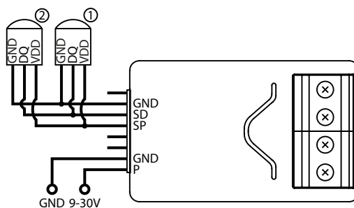
Schemat 3: Połączenie z 2 czujnikami DS18B20 (1,2 – czujnik DS18B20)
